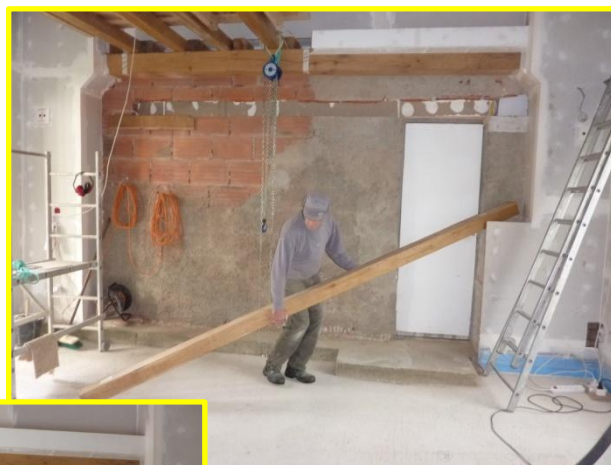
Montage et scellement de la solive séparant le petit salon et le grand salon
